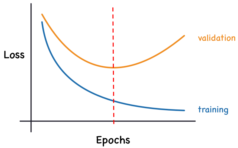
合适拟合
