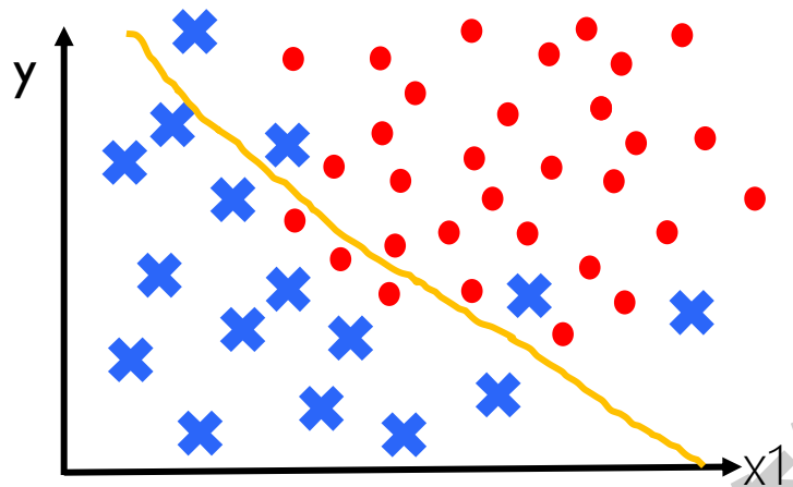
欠拟合
