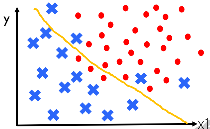
欠拟合
